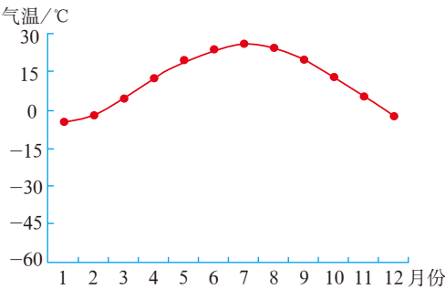
图3.12 气温年变化
