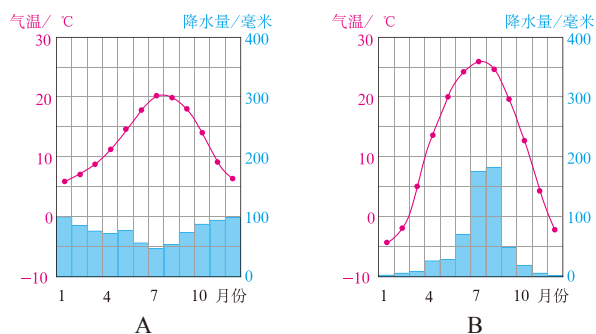
图3.26 A、B两地多年平均各月气温和降水量
