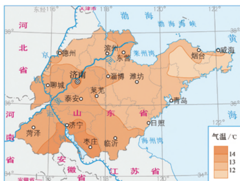
图3.31 山东省年平均气温的分布
