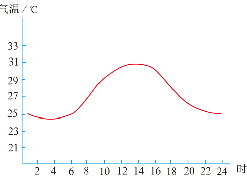
图3.11 气温日变化
