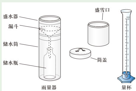
图3.21 雨量器和量杯
