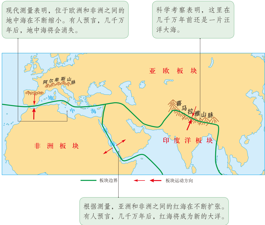
图2.24 红海、地中海、喜马拉雅山脉成因示意
