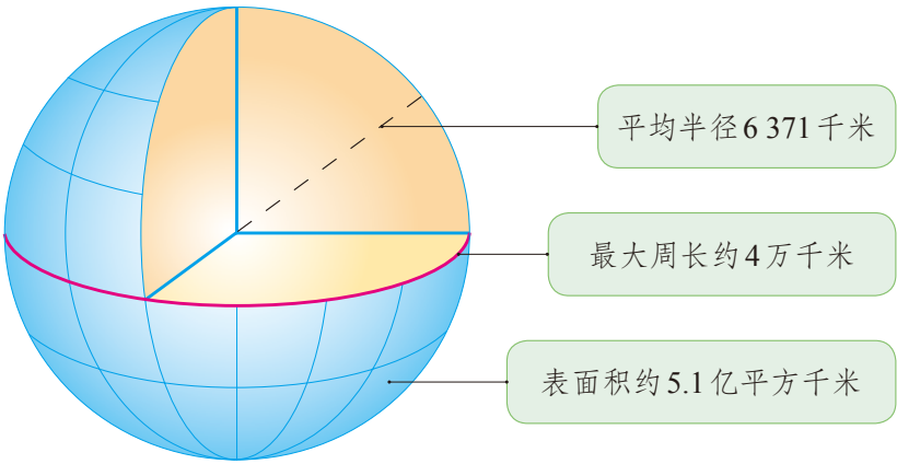
图 1.2 地球的大小
