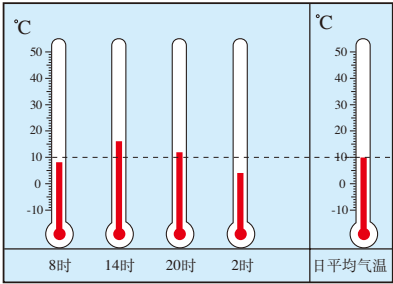
图3.10 日平均气温
