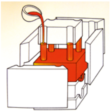
青铜器浇铸示意图（合范法）
